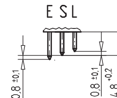
Stecklänge / mating length
