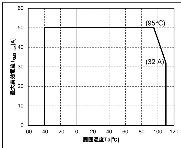
Figure 4. CQ-2232のディレーティングカーブ
