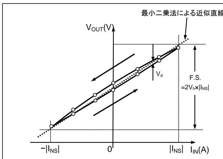
Figure 5. CQ-2232の出力特性
