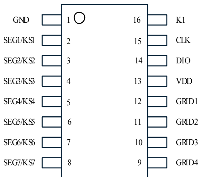
图1 管脚定义
