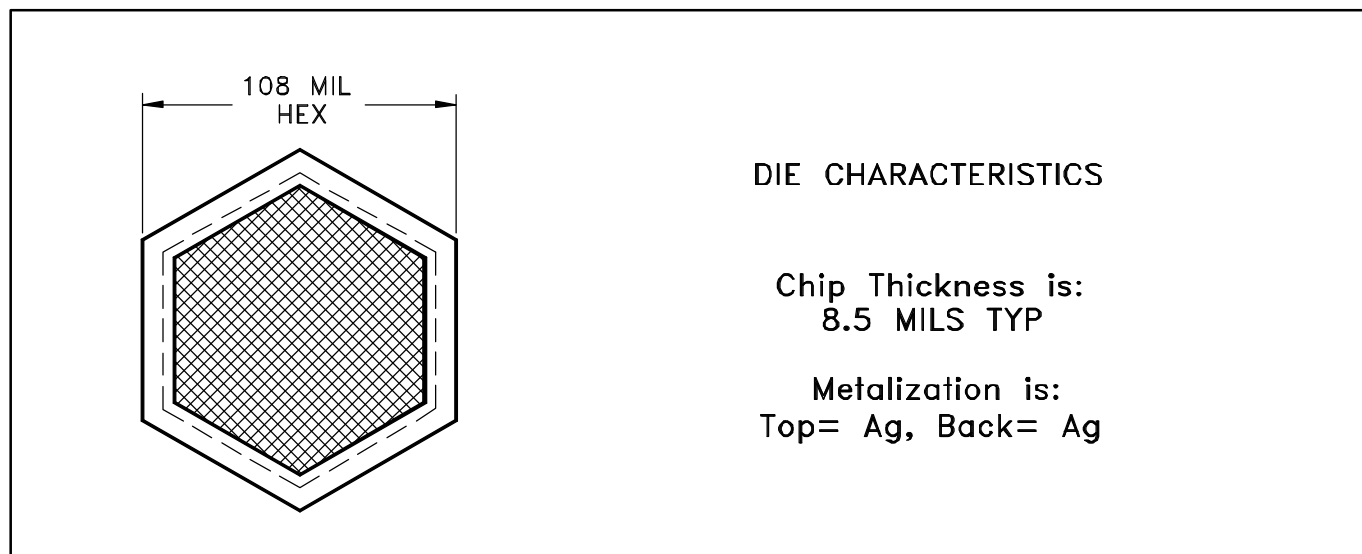
DIE OUTLINE
