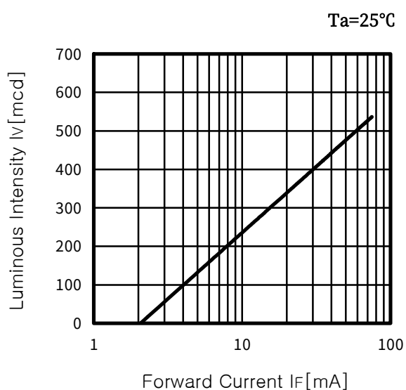
Fig. 2 I_v - I_F
