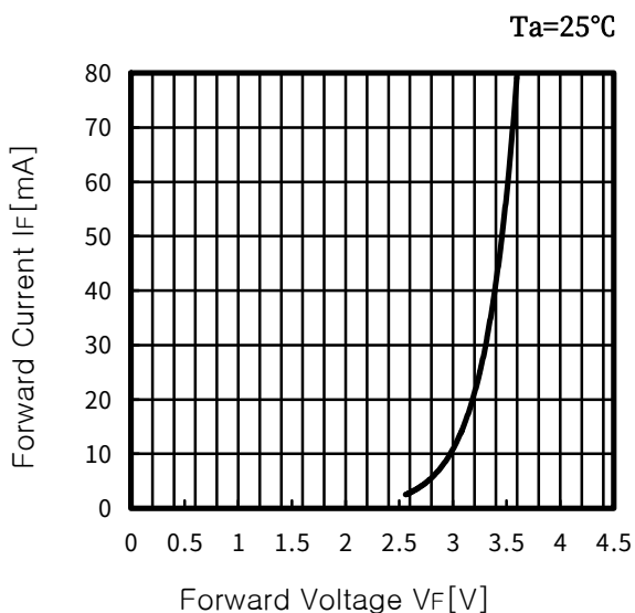
Fig. 1 I_F - V_F
