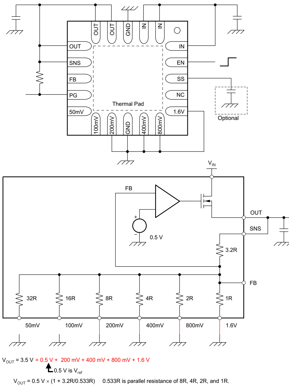
图 6-6. 3.5-V Configuration
