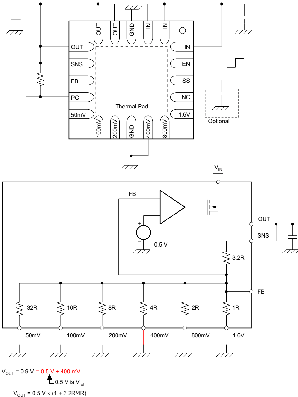
图 6-1. 0.9-V Configuration
