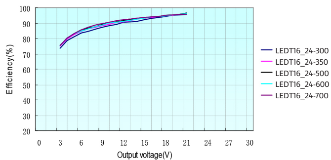
Vin=24V
