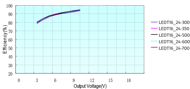
Vin=12V
