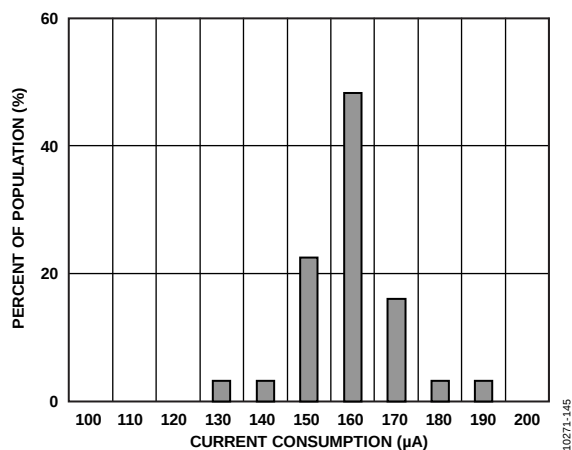
图46. 25°C时的功耗, 100 Hz输出数据速率, V_s = 2.5 V, 31个器件
