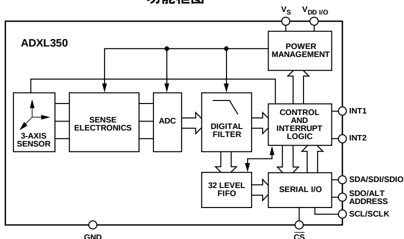
功能框图
