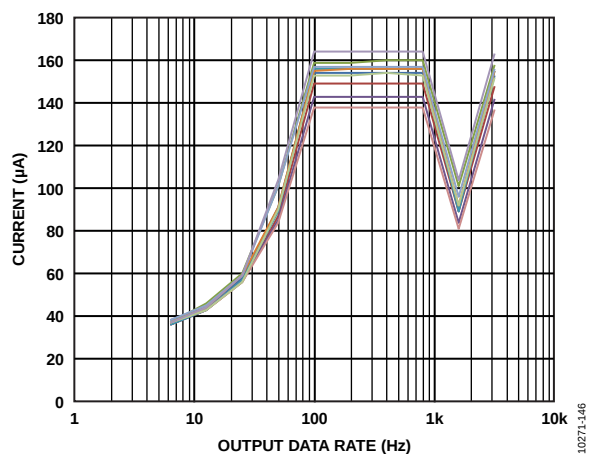
图47. 25°C时功耗与输出数据速率的关系, V_s = 2.5 V, 10个器件
