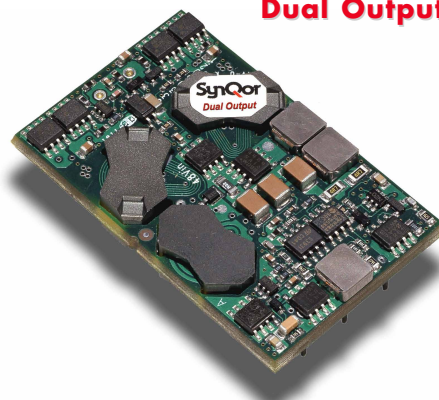
DQ61212QMA06 Module
