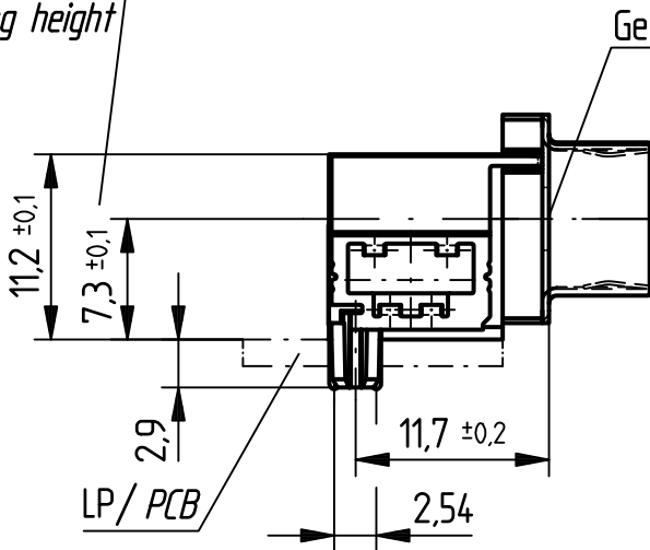
Ansicht X
