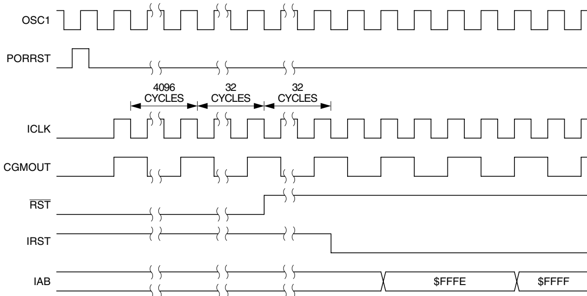
Figure 7-7. POR Recovery
