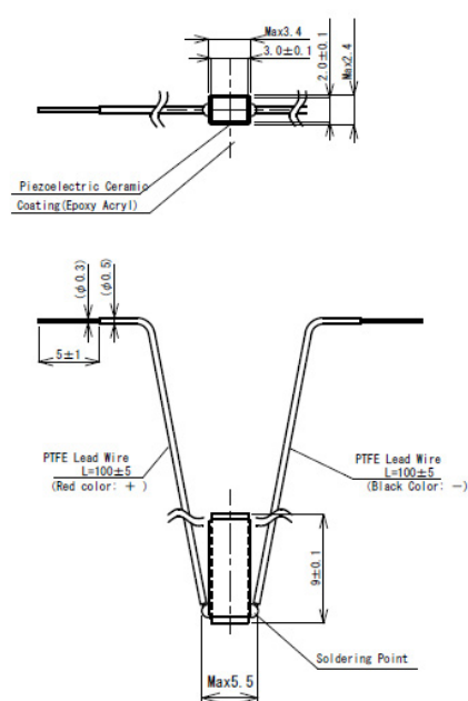
AE0203D08H09DF
