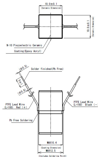
AE1010D16DF
