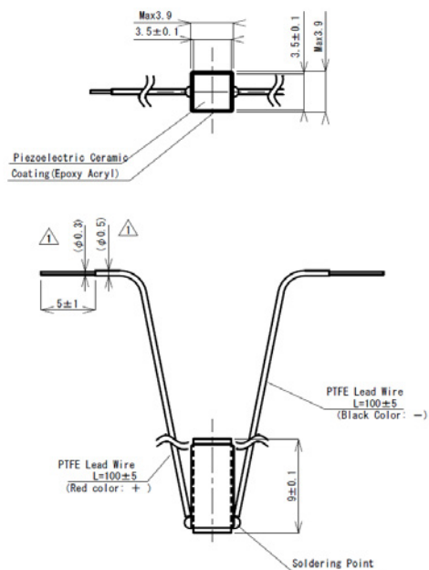
AE035035D08H09DF
