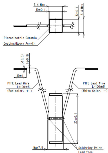
AE0505D16DF
