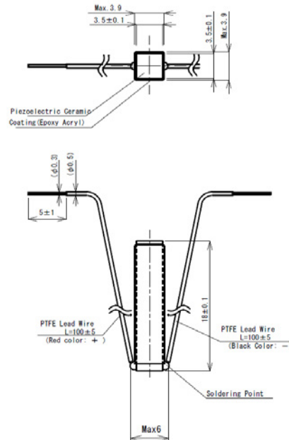
AE035035D18H18DF
