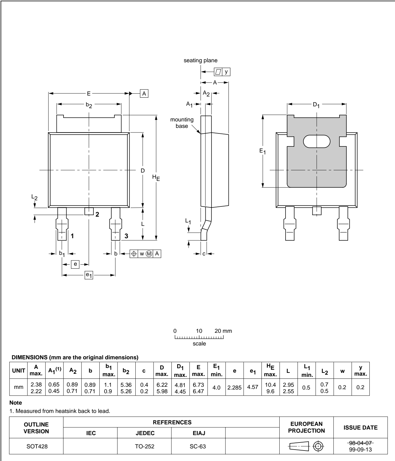
Fig 16. SOT428 (D-PAK).
