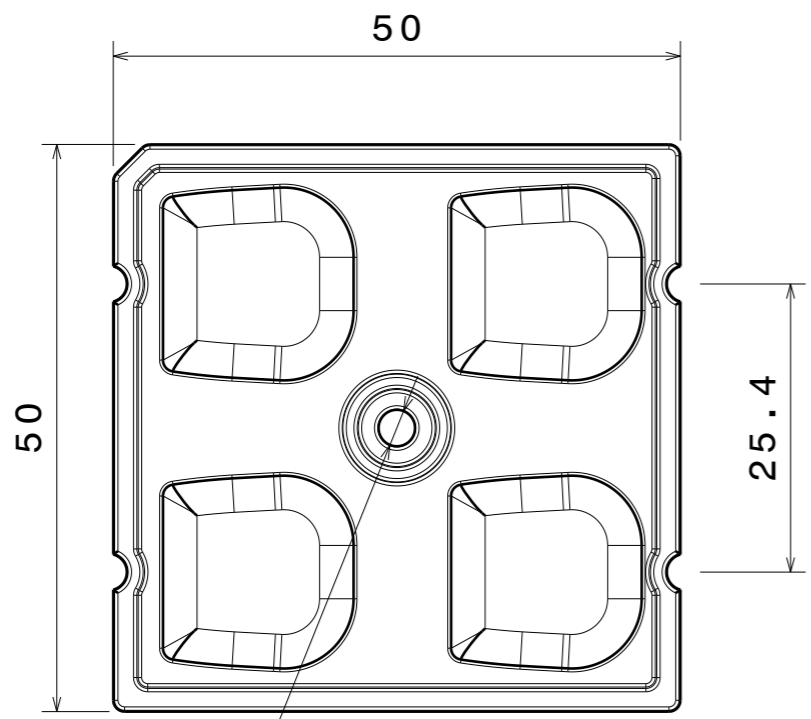
Top view Scale: 3:2
