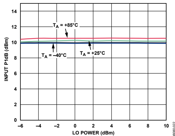
Figure 24. Input P1dB vs. LO Power
