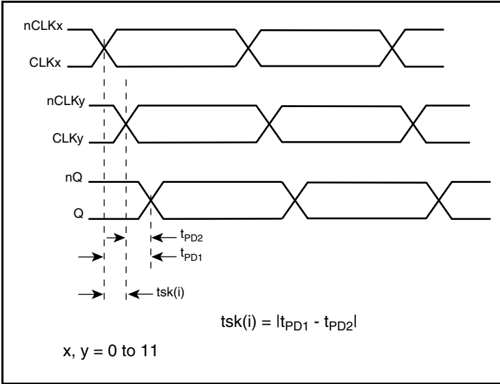
Input Skew
