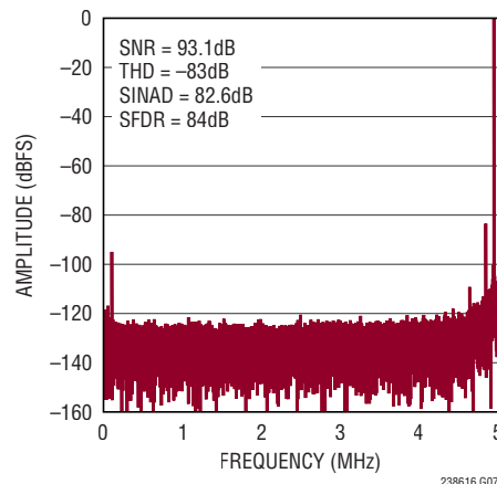
32k Point FFT f_{SAMPL} = 10\text{Mps} , f_{IN} = 5\text{MHz}
