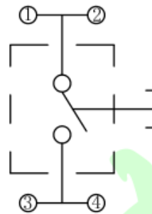
原理图
