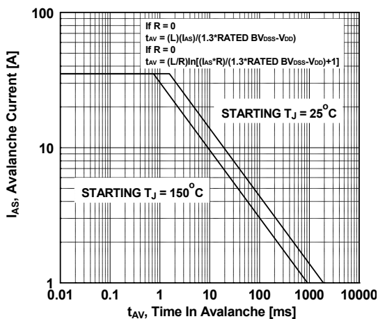
图 11. 非箝位感性开关能力
