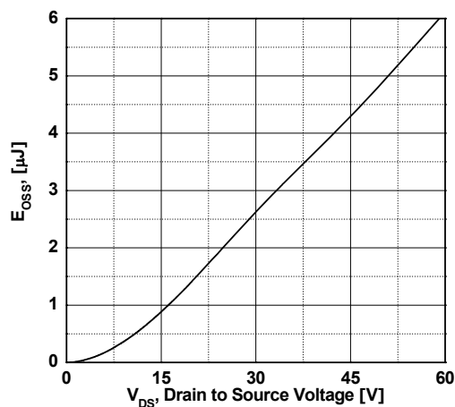
图 12. Eoss 与漏源极电压
