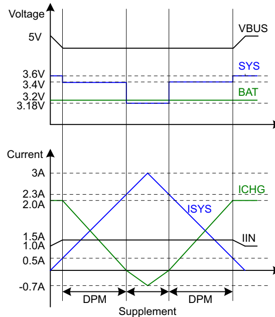
图 13. DPM Response
