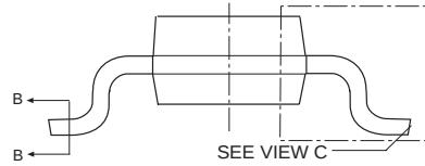
VIEW A-A
