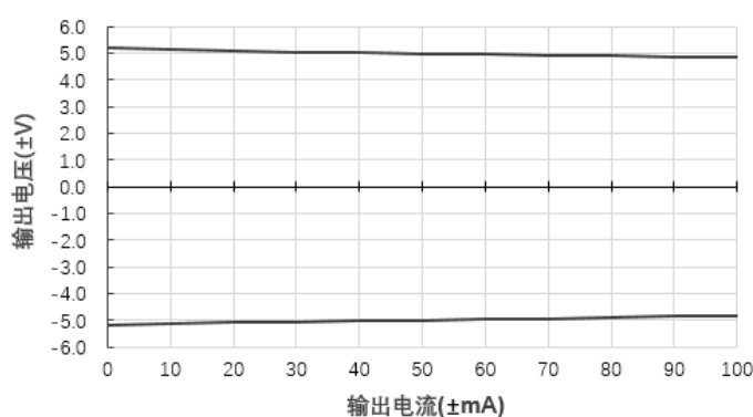
输出电压Vs输出电流(Vin=12V)@A1205S-1WR3
