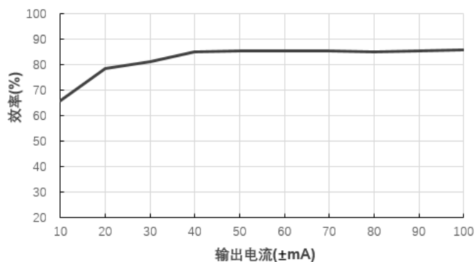
效率Vs输出电流(Vin=5V)@A0505S-1WR3
