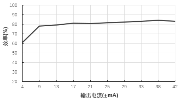
效率Vs输出电流(Vin=5V)@A0512S-1WR3
