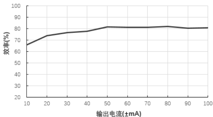
效率Vs输出电流(Vin=12V)@A1205S-1WR3
