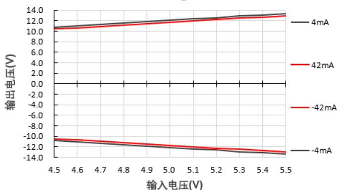
输出电压Vs输入电压@A0512S-1WR3
