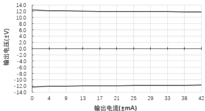
输出电压Vs输出电流(Vin=5V)@A0512S-1WR3
