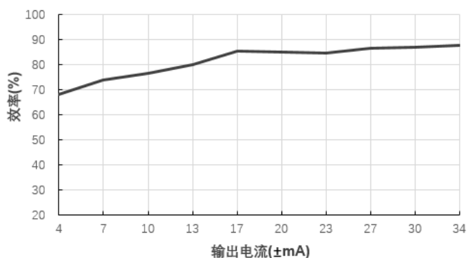
效率Vs输出电流(Vin=12V)@A1215S-1WR3
