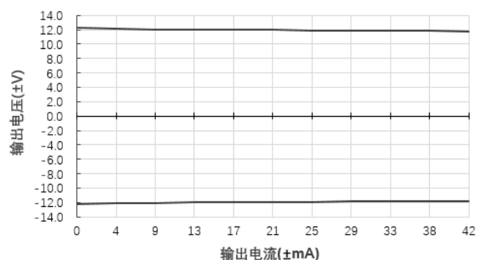
输出电压Vs输出电流(Vin=12V)@A1212S-1WR3
