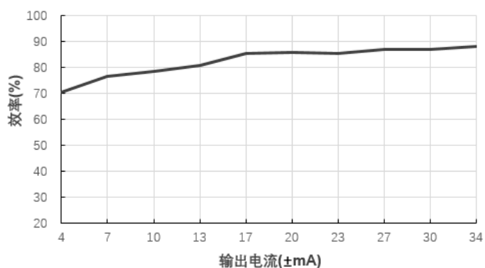
效率Vs输出电流(Vin=12V)@A1212S-1WR3
