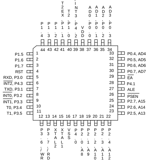
44-Pin QFP (W78LE58F)
