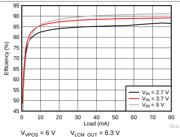
图 197. VPOS Efficiency
