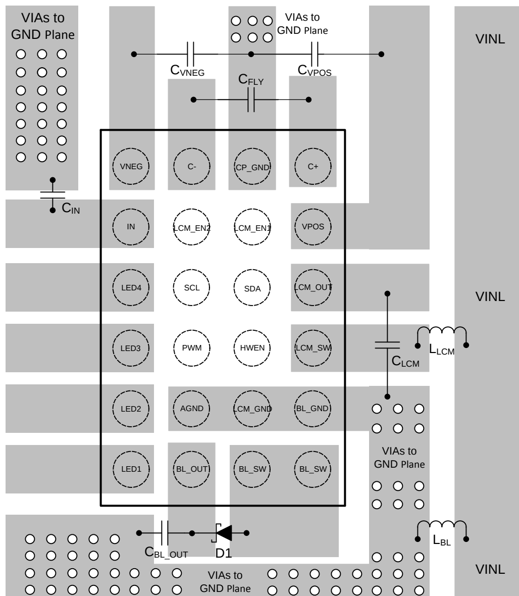
图 211. LM36274 Layout Example
