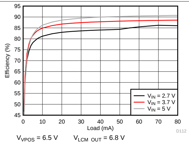
图 198. VPOS Efficiency
