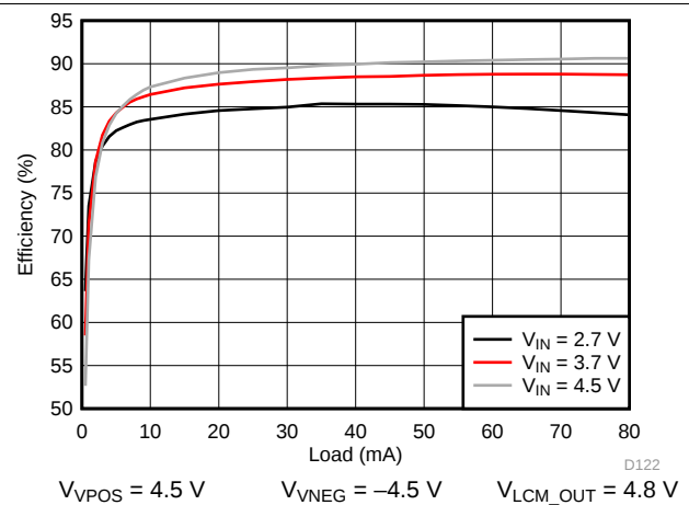
图 208. VPOS/VNEG Efficiency
