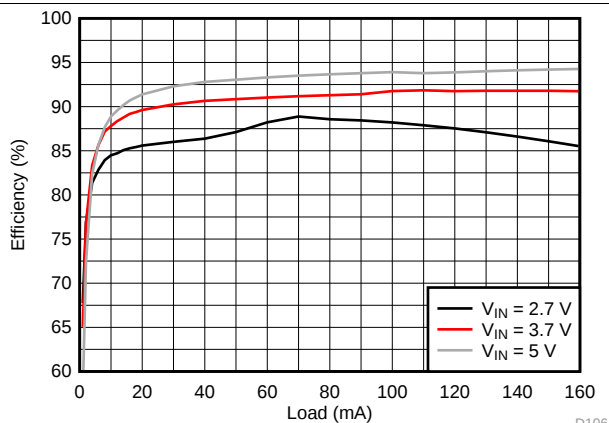
图 190. LCM Boost Efficiency
