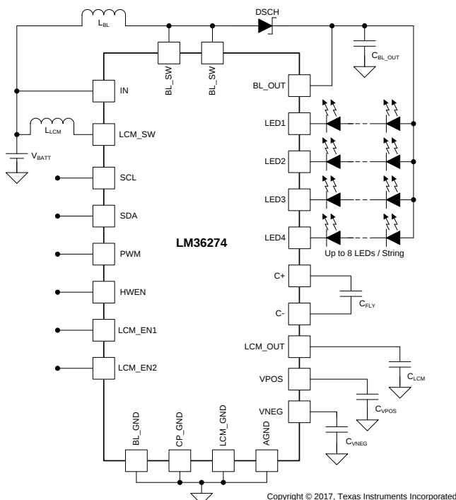
简化原理图
