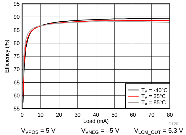
图 206. VPOS/VNEG Efficiency
