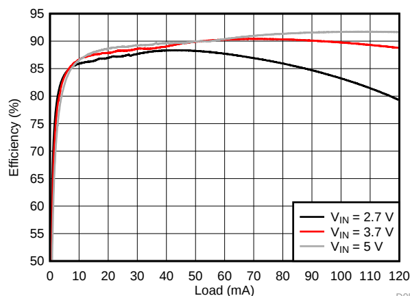
背光效率, 4P6S
