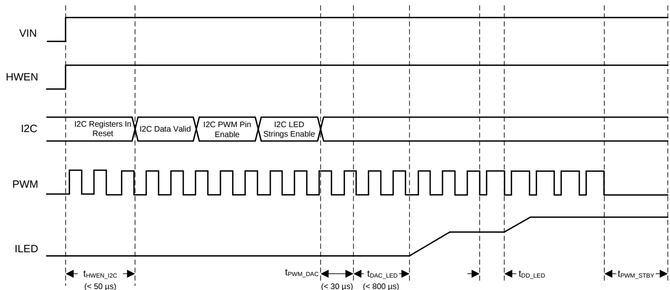
图 32. Enabling the LM36274 via PWM
