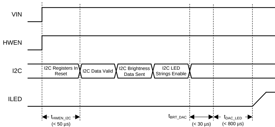
图 31. Enabling the LM36274 via I 2 C
