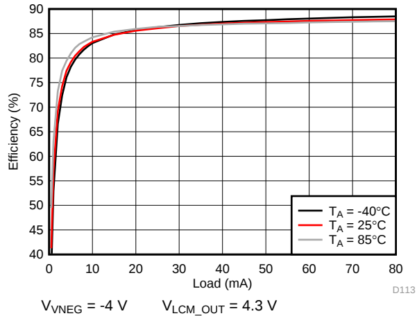
图 199. VNEG Efficiency
