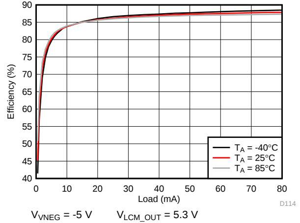
图 200. VNEG Efficiency
