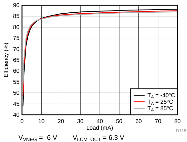
图 201. VNEG Efficiency
