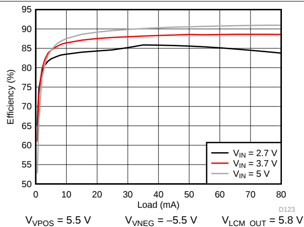
图 209. VPOS/VNEG Efficiency
