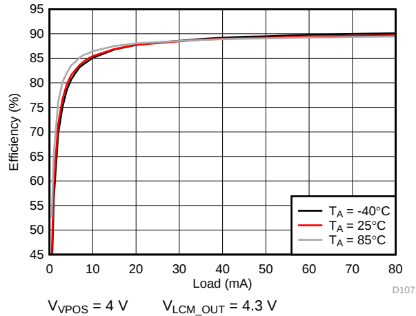
图 193. VPOS Efficiency
