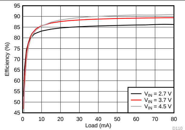
图 194. VPOS Efficiency
