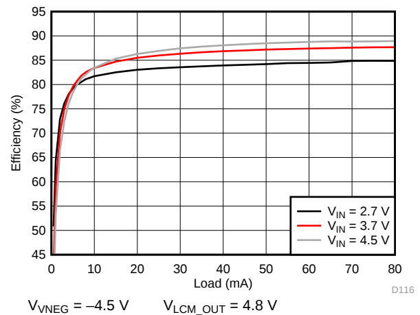
图 202. VNEG Efficiency
