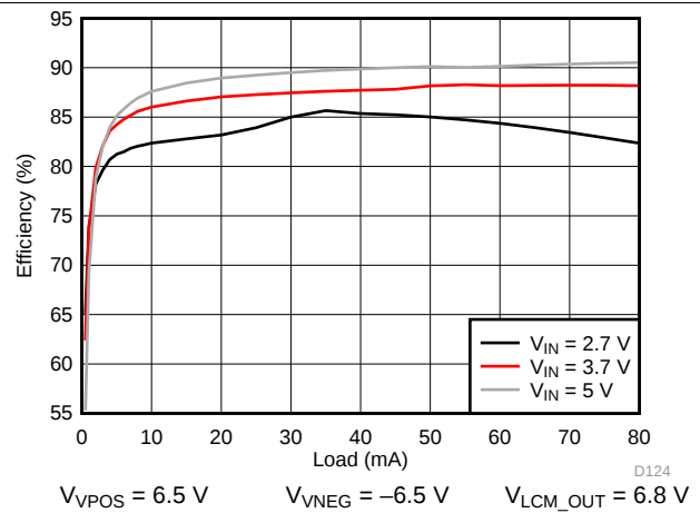
图 210. VPOS/VNEG Efficiency
