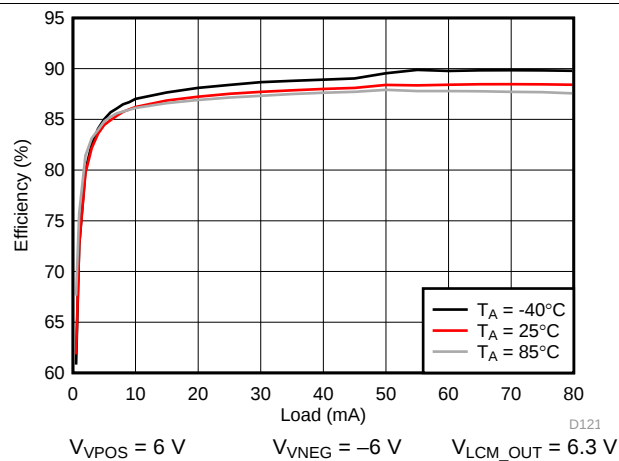
图 207. VPOS/VNEG Efficiency
