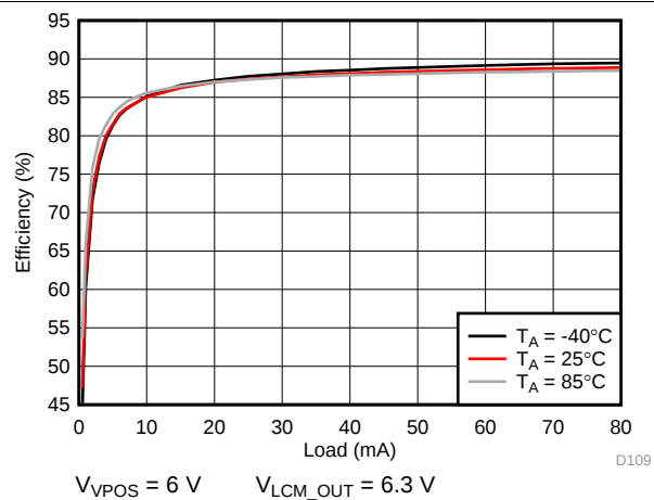
图 195. VPOS Efficiency
