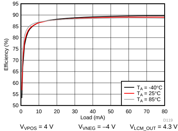
图 205. VPOS/VNEG Efficiency
