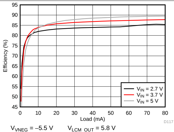
图 203. VNEG Efficiency
