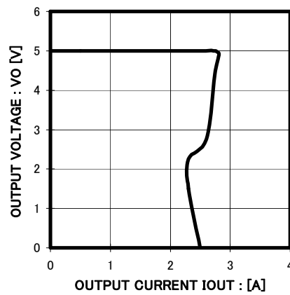
Fig.2 OCP VCC=20V
