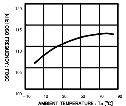
Fig.12 fosc-Ta
