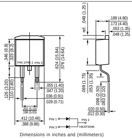
D2-PAK
