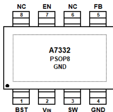
PSOP8, P8
