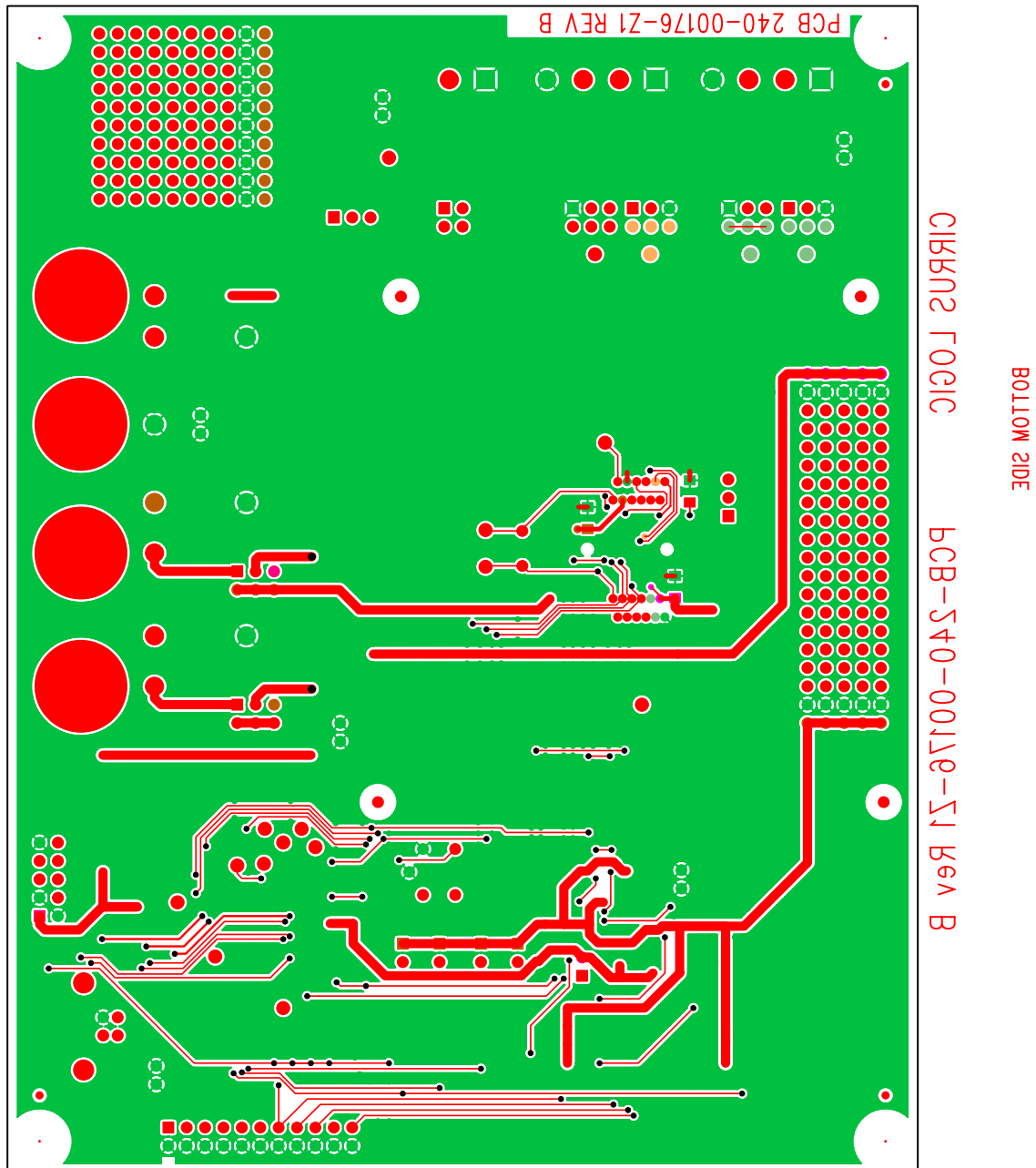
Figure 24. Bottomside Layer
