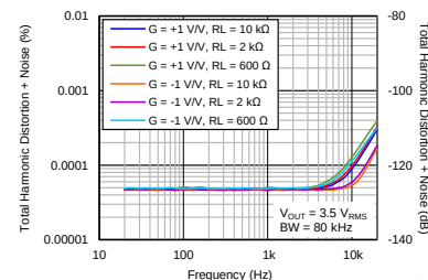
出色的总谐波失真 (THD) 性能
