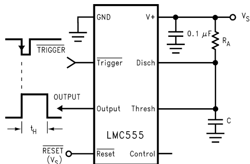
图 11. 单稳（一次性）
