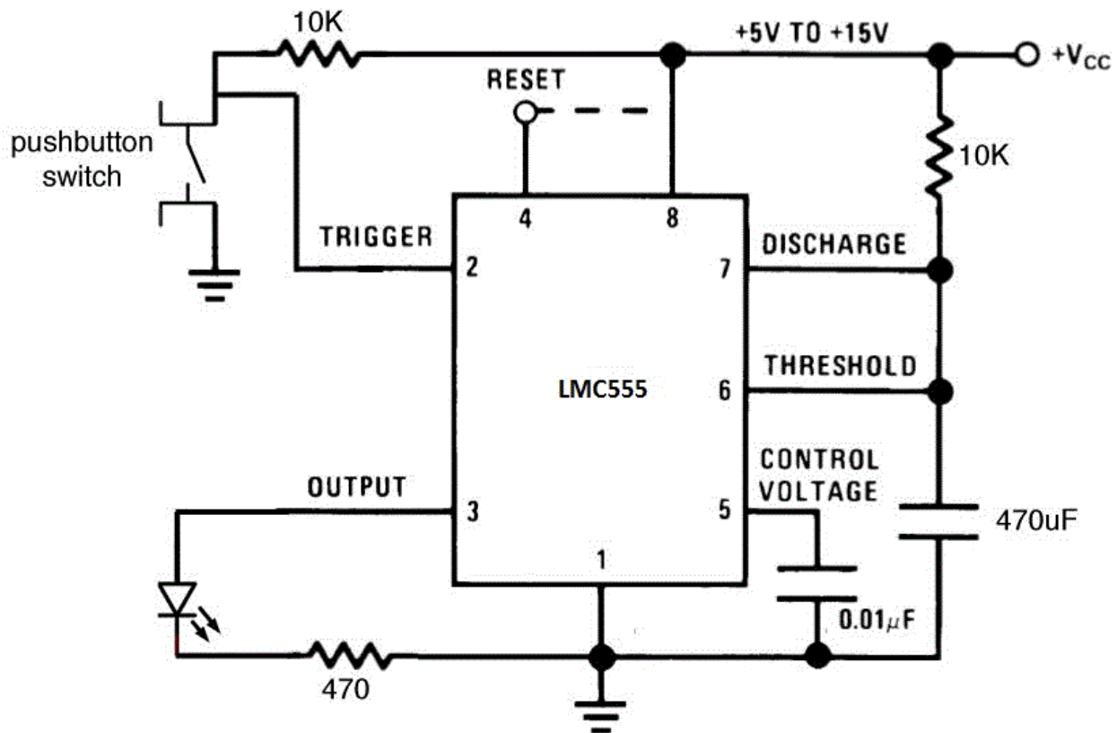
图 9. 在单稳模式下闪烁 LED 的原理图
