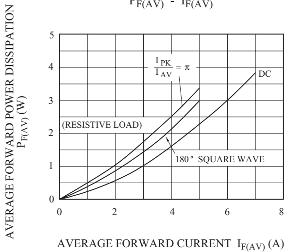
P_{F(AV)} - I_{F(AV)}
