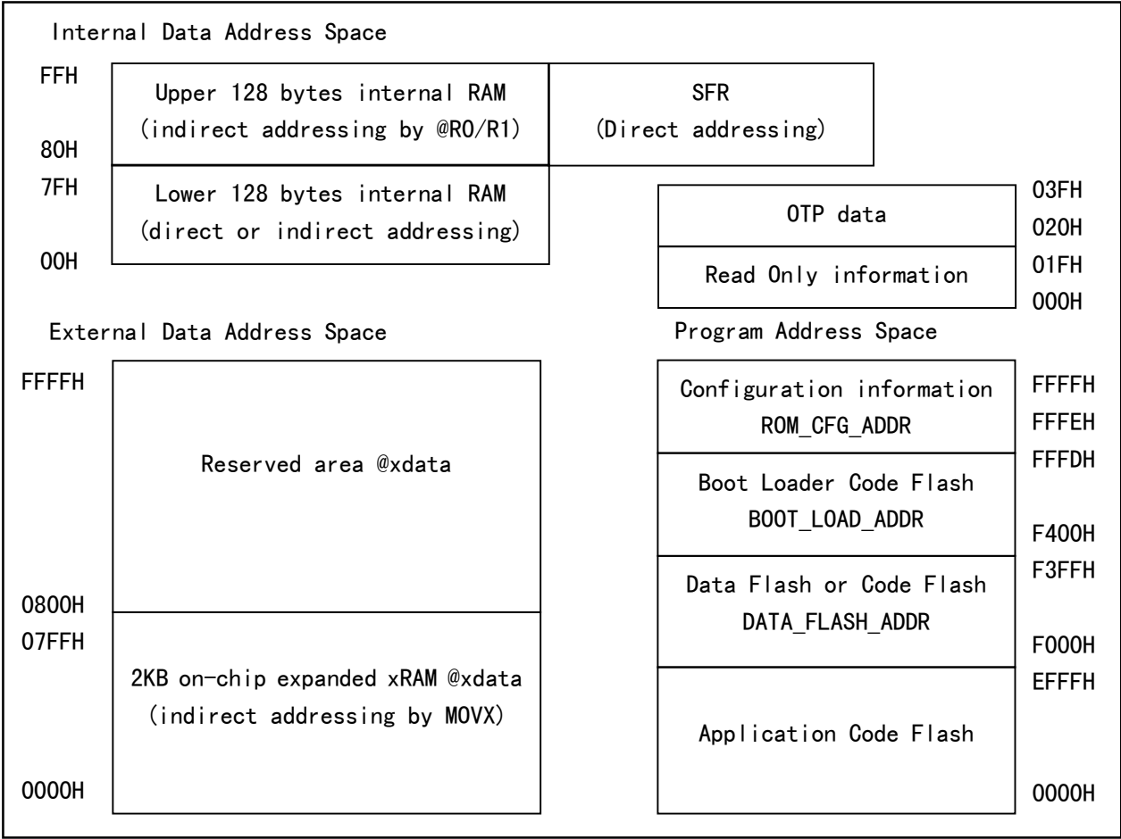
CH549 寻址空间分为程序存储空间、内部数据存储空间、外部数据存储空间、只读和 OTP 空间。 图 6.1 存储器结构图
