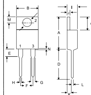
TO-220A
