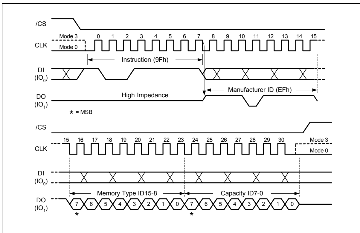
Figure 25. Read JEDEC ID
