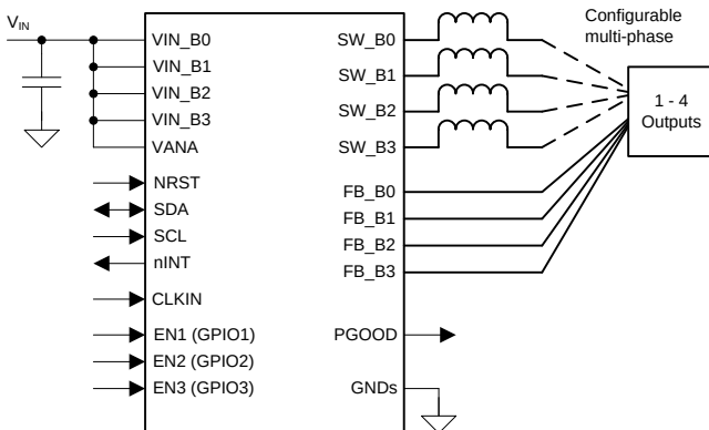
简化原理图
