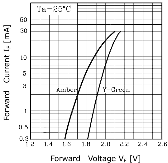
Fig. 1 I_F - V_F
