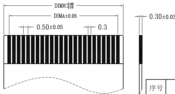
适用扁平线
