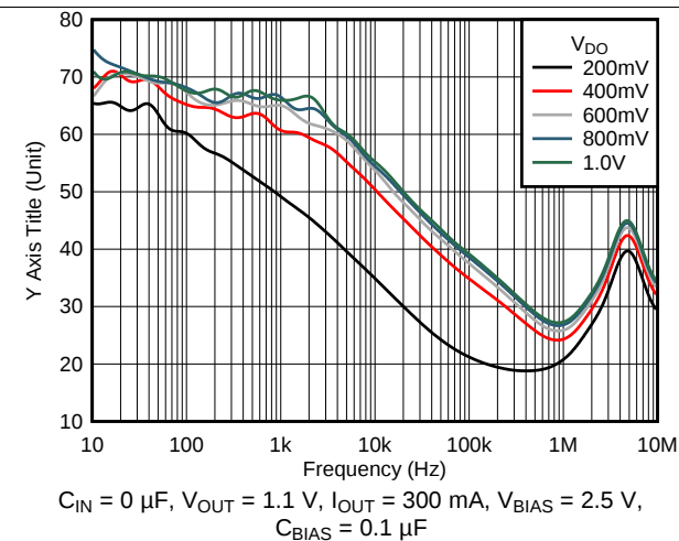
图 29. PSRR vs Frequency and V_{DO}
