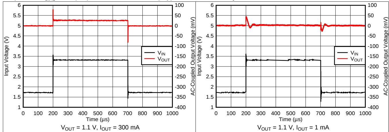
图 13. V_{IN} Transient
