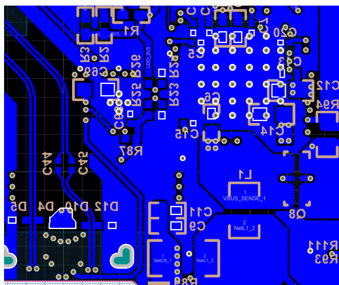
图 12-11. Bottom Layer Component Routing
