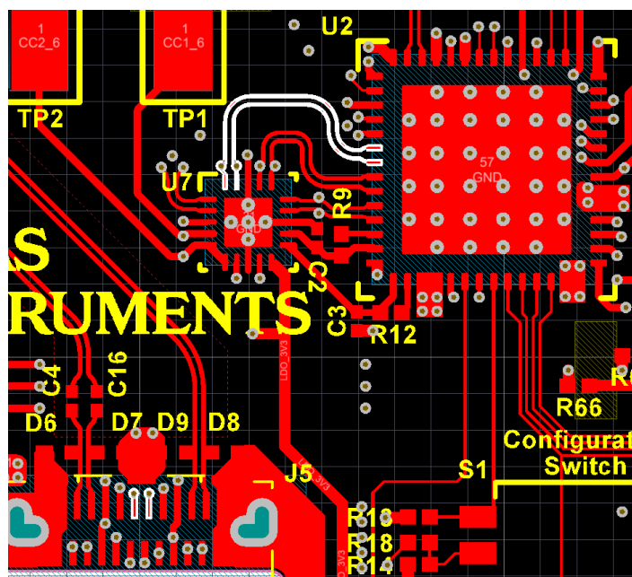
图 12-10. Top Layer Component Routing
