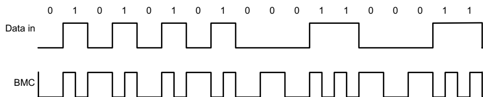
图 9-4. Biphas Mark Coding Example
