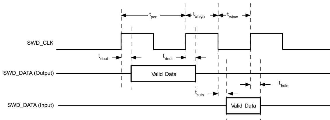
图 8-6. SWD Timing
