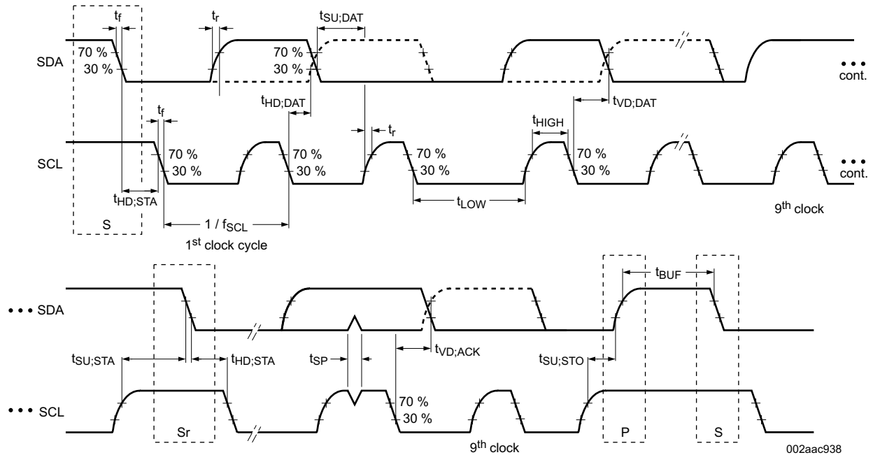
图 8-4. I²C Slave Interface Timing
