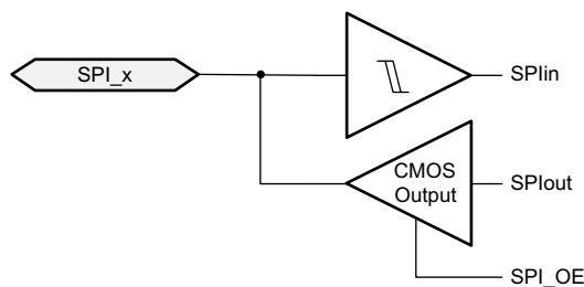
图 9-50. IOBUF_GPIOHSSI
