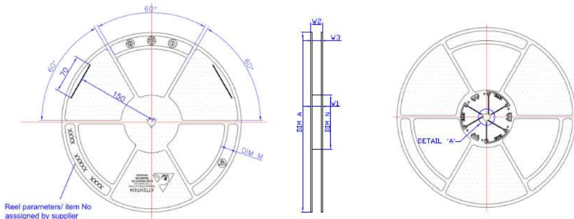
DML1006LDS-13
