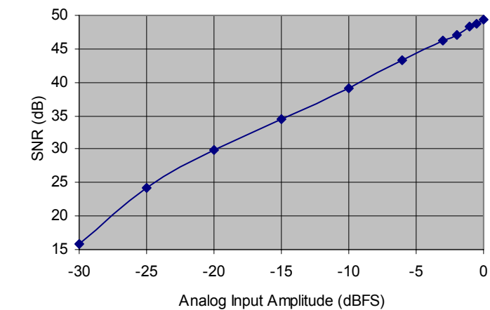
Figure 3. SNR vs. Vin
