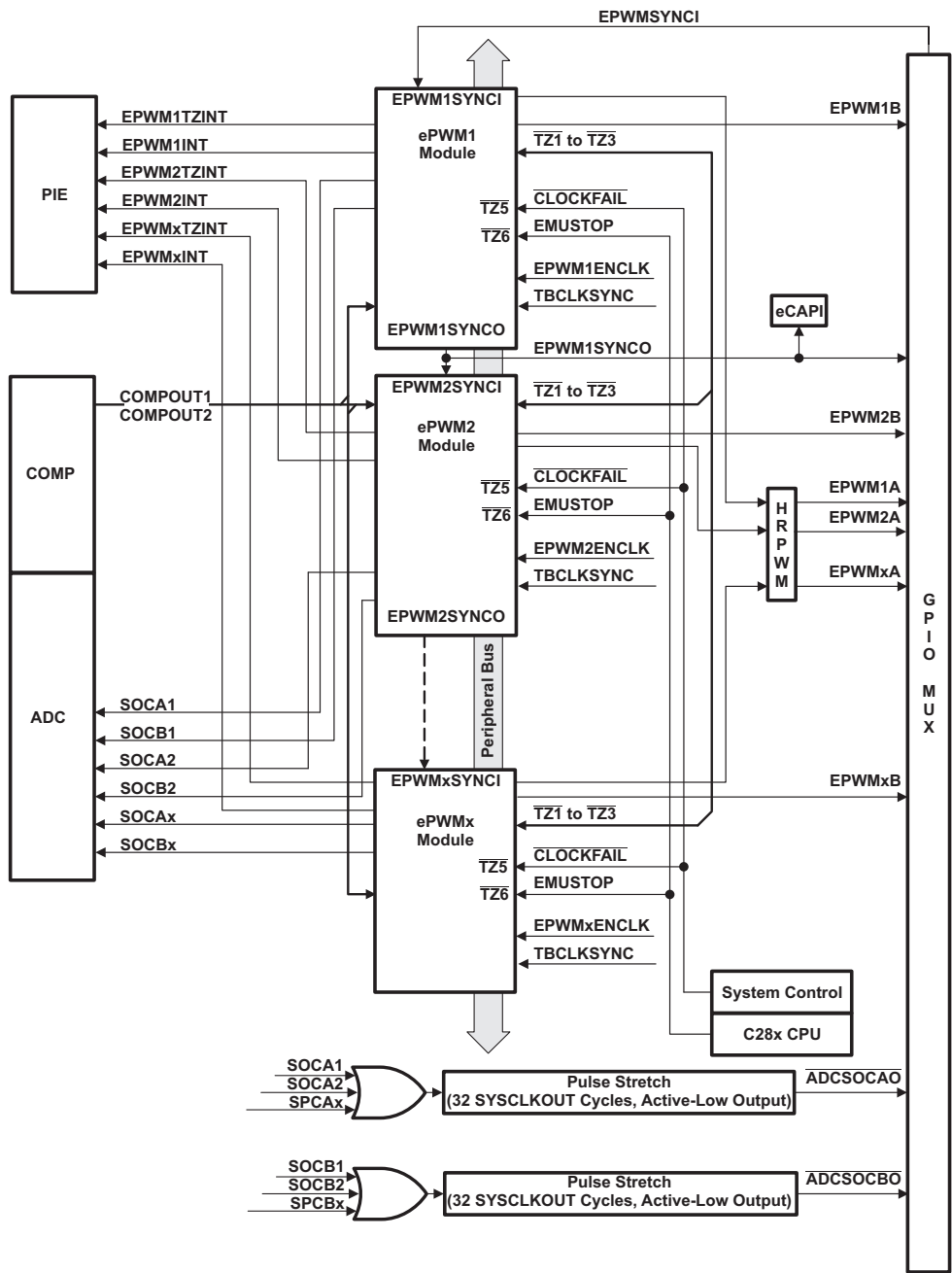
图 4-8. ePWM
