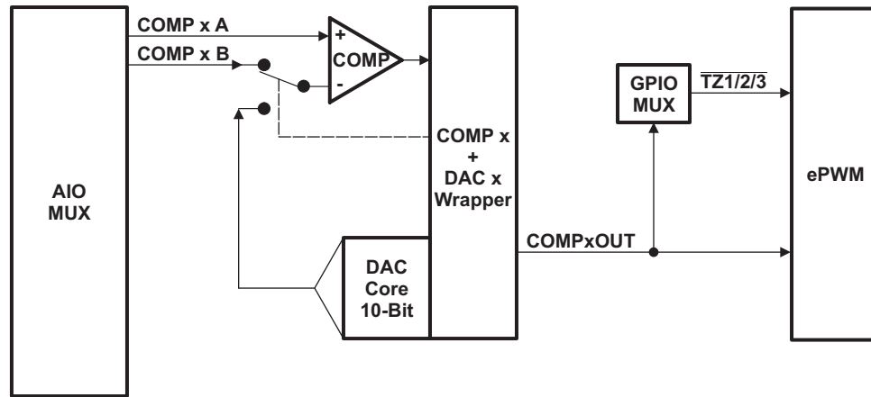
图 4-4. 比较器块图
