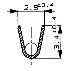
断面 C-C (SECT. C-C)
