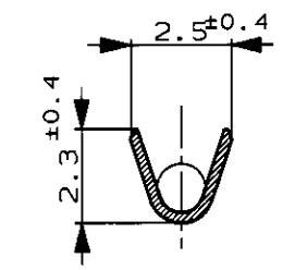
断面 B-B (SECT. B-B)
