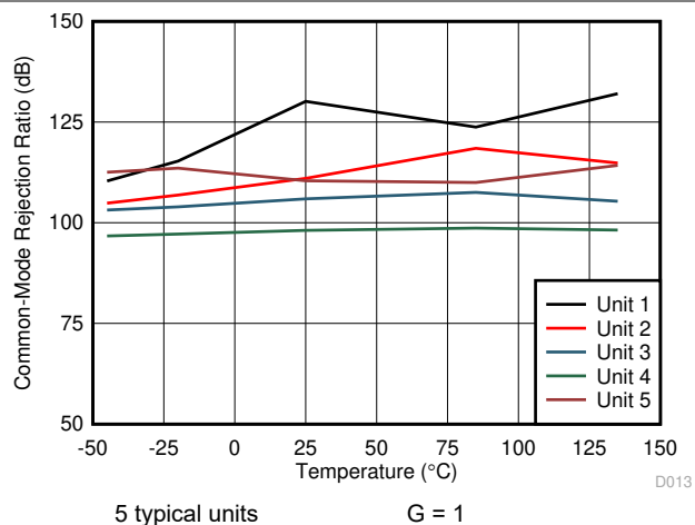
图 7-14. CMRR vs Temperature
