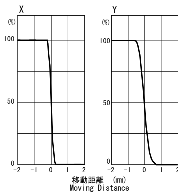
■ 位置検出特性 *2 相対 I_C /移動距離
