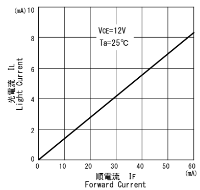
■ 光電流/順電流特性 I_C/I_F
