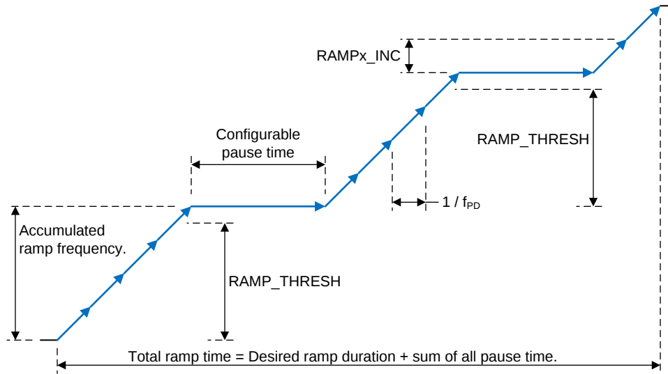
图 173. Auto Ramp Waveform
