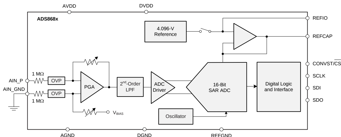
方框图
