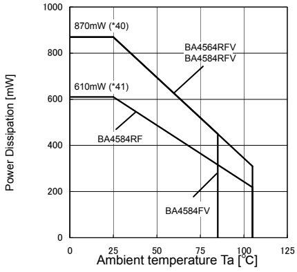
(d)BA4564R/BA4584/BA4584R family
