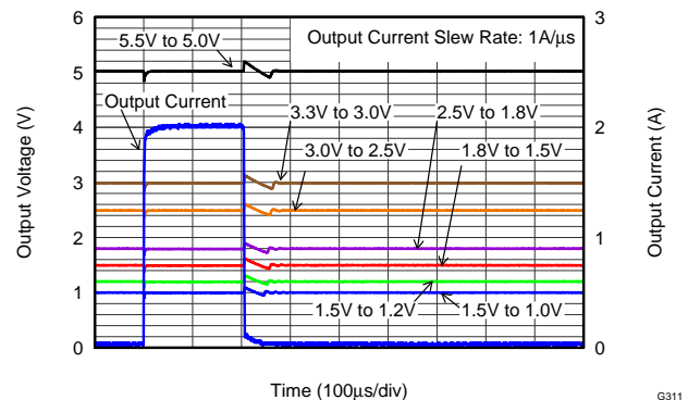
负载瞬态响应 (7 种不同输出)
