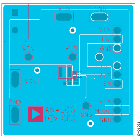
Figure 37. Top Layer
